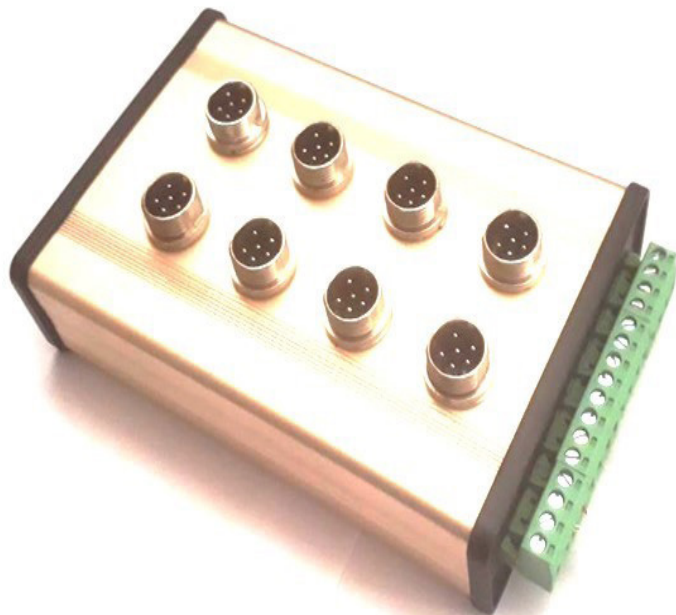
شکل ۳: دیتالاگر دمای ۸ کاناله RTD و ۸ کاناله ترموکوپل [1]
