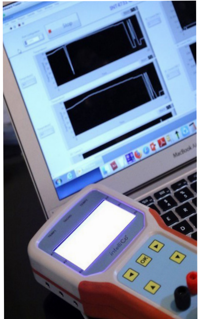
شکل ۲: یک نمونه از دیتالاگرهای دما که خروجی را به صورت آنلاین در نمایشگر روی دیتالاگر و در نرم‌افزار لب ویو نمایش می‌دهد [1]
