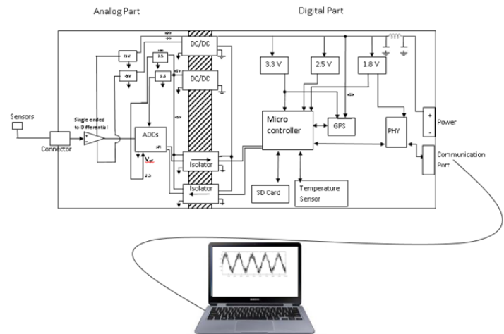
شکل ۵: بلوک دیاگرام یک دیتالاگر با قابلیت اتصال حسگرهای شتاب پیزو (IEPE) و به صورت ایزوله [4]
