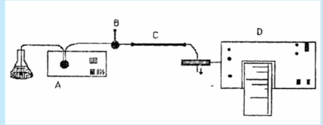
شکل ۱: نمای ساده از کروماتوگرافی مایع با کارایی بالا. بخش‌های مختلف به ترتیب حروف مشخص شده‌اند: پمپ، محل تزریق، ستون و آشکارساز [۱۴]
