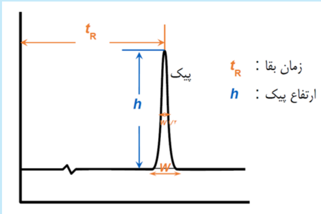
شکل ۲: نمای یک کروماتوگرام. محور افقی معرف زمان و محور عمودی درصد غلظت ترکیب را مشخص می‌کند [۱۶].
